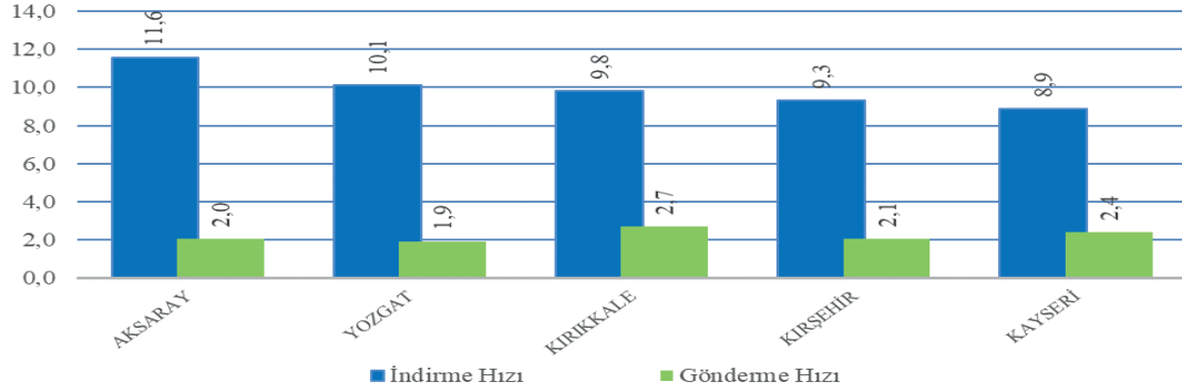
Şekil 3-7 Mobil Veri İndirme ve Gönderme Hızları (Mbps)
